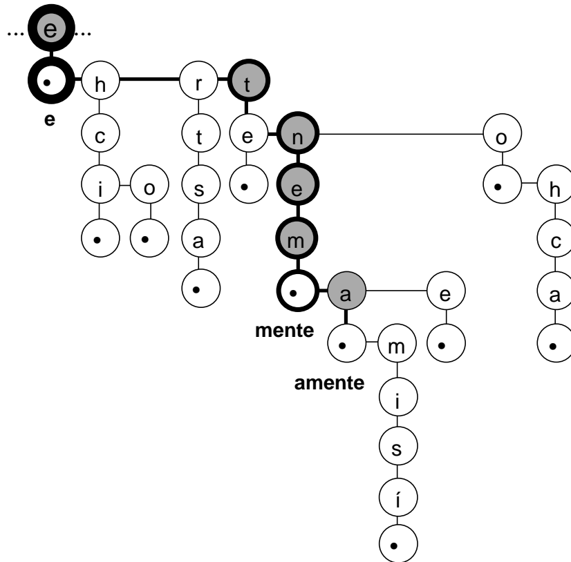
Figura 4: Árbol de terminaciones
